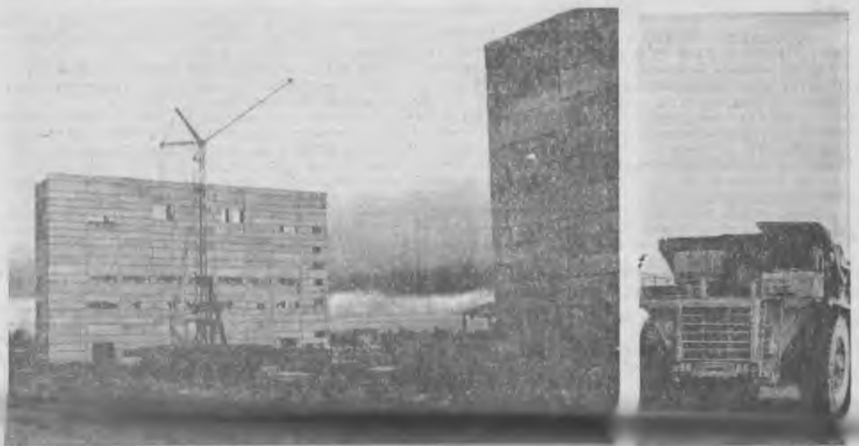
В октябре активно продолжались общестроительные и монтажные работы на объектах будущего щебеночного завода. Закончена сборка горизонтальной части галереи конвейера № 1, которая соединит корпус крупного дробления и промежуточный бункер. В начале ноября будет проведен монтаж. На корпусе грохочения смонтированы железобетонные перекрытия. Строятся инженерные коммуникации: теплосети и пультопровода.
