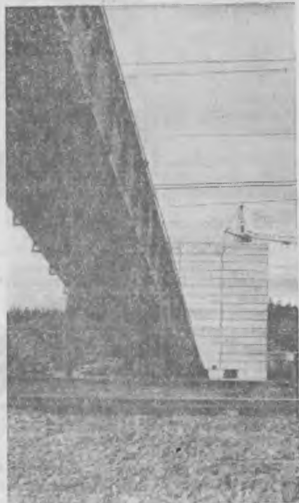
В октябре активно продолжались общестроительные и монтажные работы на объектах будущего щебеночного завода. Закончена сборка горизонтальной части галереи конвейера № 1, которая соединит корпус крупного дробления и промежуточный бункер. В начале ноября будет проведен монтаж. На корпусе грохочения смонтированы железобетонные перекрытия. Строятся инженерные коммуникации: теплосети и пультопровода.
